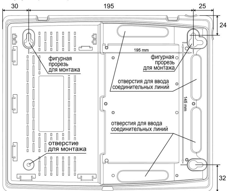
Рис.3 Задняя стенка прибора. Присоединительные размеры
