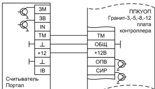
Рис.Б5 Схема подключения считывателя «Портал»
