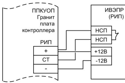
Рис.Б6 Схема подключения источника внешнего электропитания резервированного (РИП)
